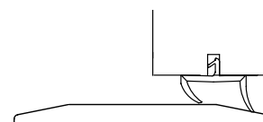
Skrå terskel med slepelist Denne varianten fåes ikke till finert karm i Prosjekt-Expressortimentet.
